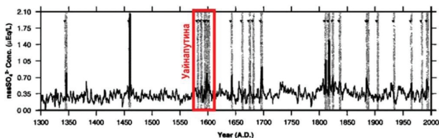
Рис. 11. Двухлетняя сглаженная запись \text{nss SO}_4 (1301–1995 гг. н. э.) и вулканические события. Красный прямоугольник – извержение Уайнапутины в 1600 г.
