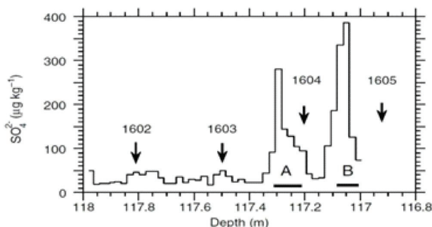
Рис. 12. Посезонные данные о концентрациях сульфатов в ледяном керне GISP2 (Гренландия, Greenland Ice Sheet Project 2) за период 1601–1605 гг. н. э.
