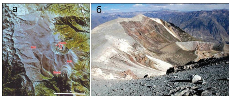
Рис. 9. а – вулкан Уайнапутина (Перу). Вид из космоса; б – и с поверхности. Видны огромные отложения пепла к западу от кратера вулкана.
