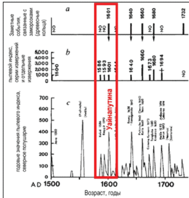
Рис. 13. «Морозные» кольца в соснах на западе США (Сьерра-Невада) и связь с крупными извержениями вулканов в глобальном масштабе.
