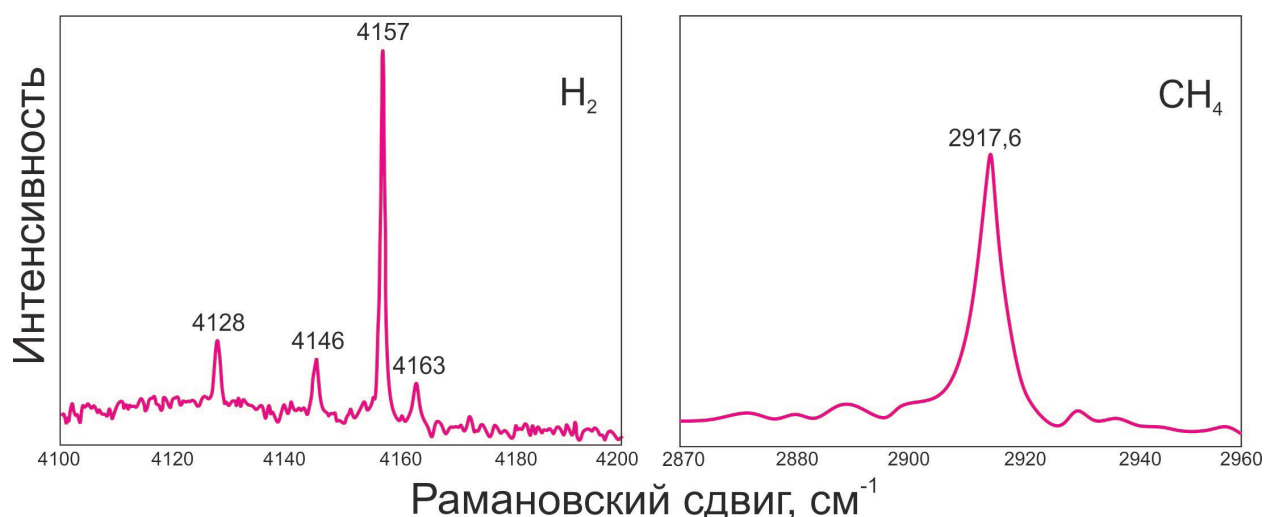
Рис. 4. Раман-спектры дочерних фаз: водорода и метана во включениях в оливине дунитов массива Матыскен. Fig. 4. Raman-spectra of the daughter phases: hydrogen and metan in inclusions in olivine from dunites of the Matysken massif.
