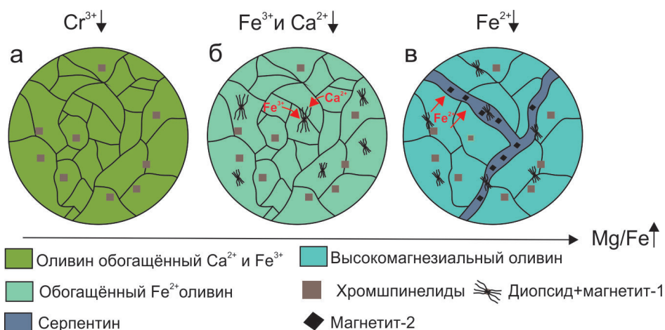
Рис. 6. Стадийность в формировании высокомагнезиального (Fo 95-96 ) оливина через серию распадов твёрдых растворов. а – распад высокобарного оливина с выделением хромшпинелидов (предположительно – магнезиоферрита), б – выделение на хромитовых зародышах диопсида и магнетита-1 (выделяется железо (3), в – серпентинизация с окислением железа (2) и выделением изометричных кристаллов магнетита-2.
